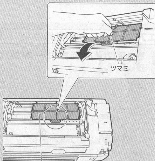
光触媒集塵・脱臭フィルター
